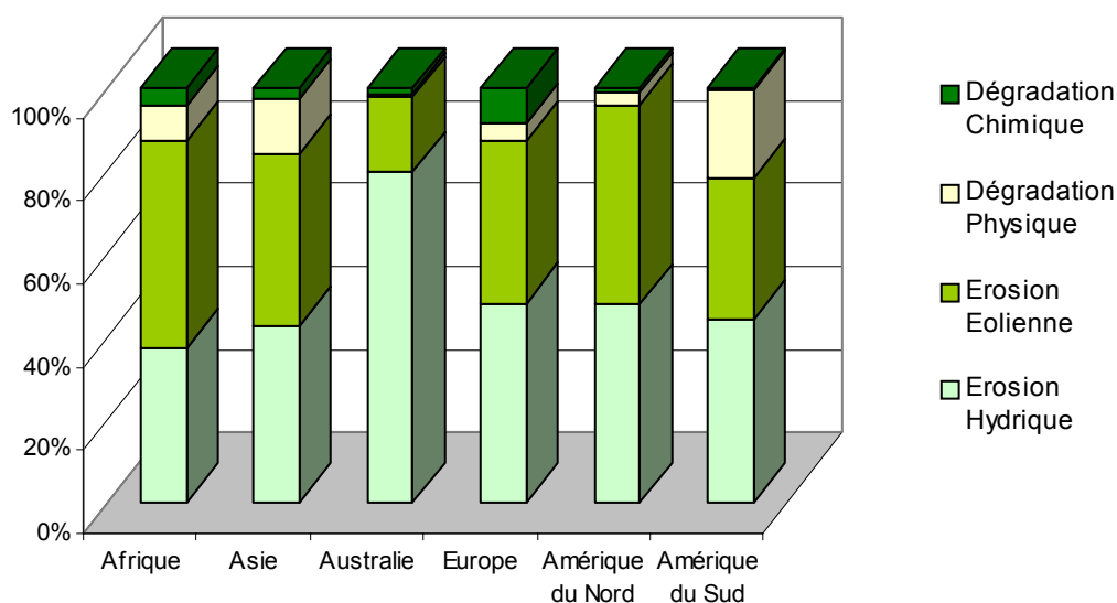
Distribution des surfaces affectées par la dégradation des sols
